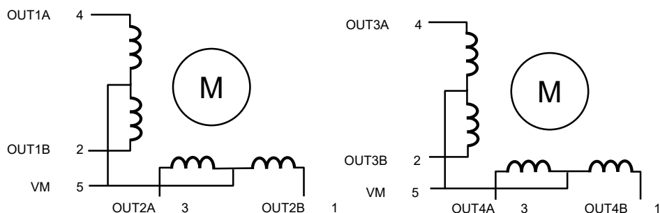
四相五線步進馬達連接圖
