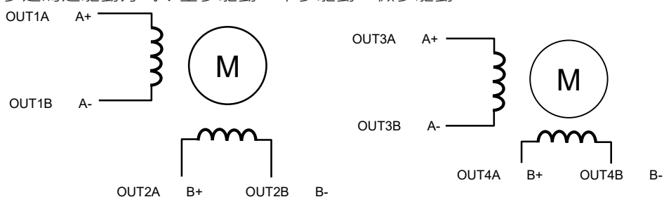
兩相四線步進馬達連接圖
